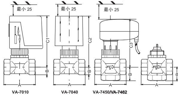
尺寸(mm)
